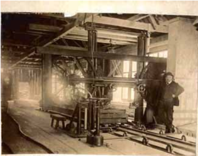
Eine Hofzonal-Bandsäge im Inneren der Sägerei (1914)
